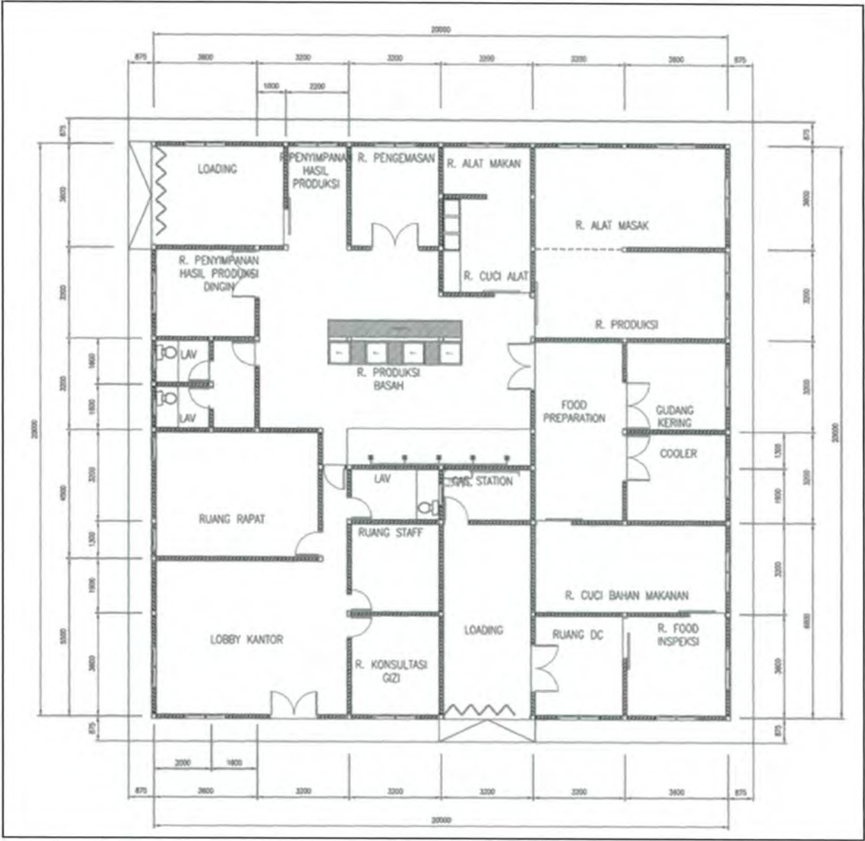
Layout Bangunan SPPG Baru dengan Luas 400 m2
